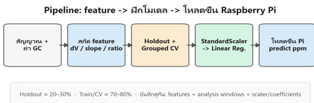
รูปที่ 13: Pipeline จากสกัด feature การแยก holdout/Grouped CV การฝึก StandardScaler–Linear Regression และการโหลดขึ้น Raspberry Pi
